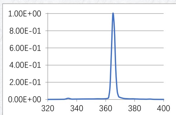
图 1. 黑光型高压汞灯的相对光谱功率分布
